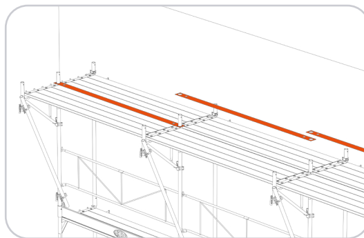
Spaltabdeckung für Gerüstkonsolen
