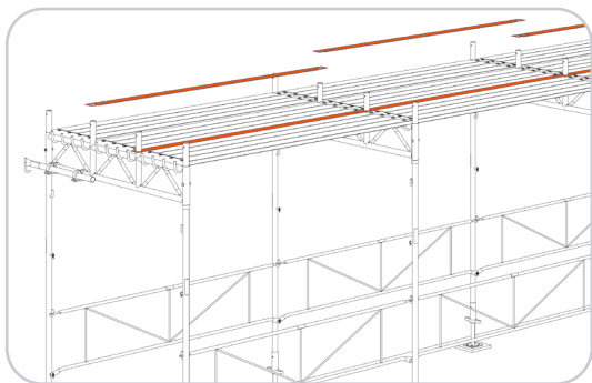
Spaltabdeckung für Passagenrahmen
